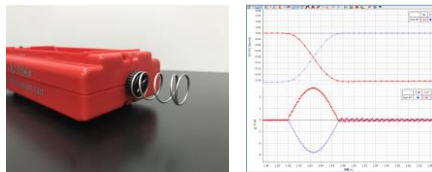
ばね同士の衝突
